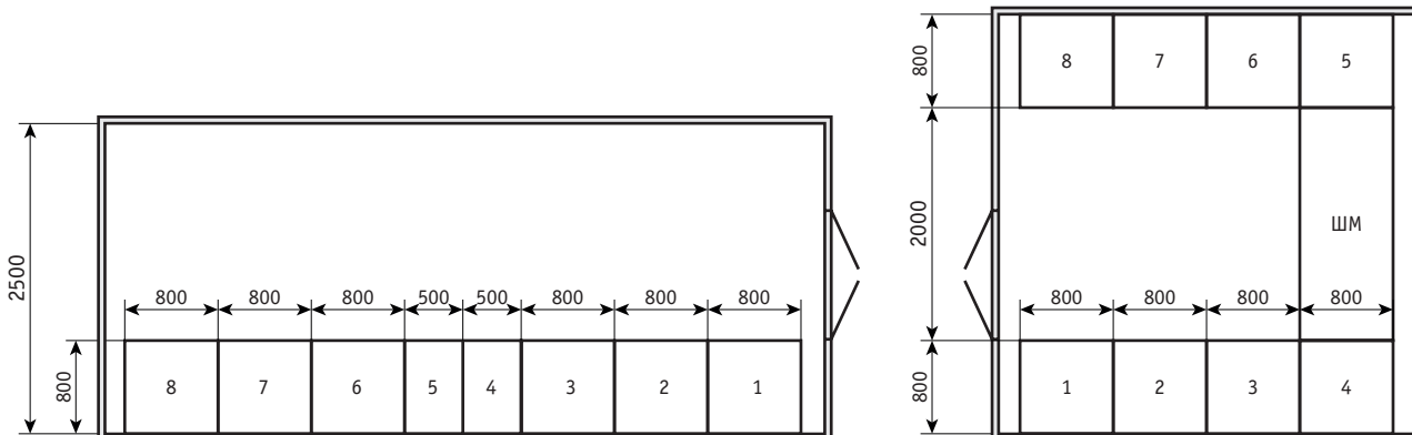
Примеры компоновки РУ 10 кВ
