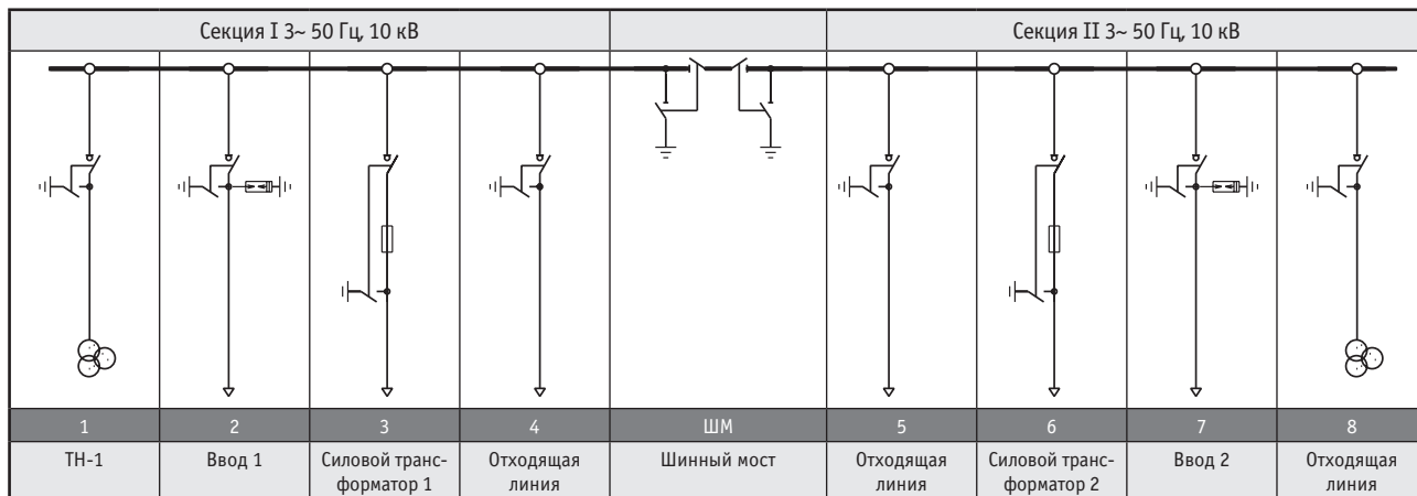
Примеры построения схем главных цепей РУ 10 кВ
